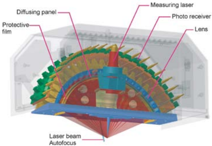
带有激光装置的阵列角度传感器
